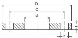
面座付さし込み溶接フランジ FF
