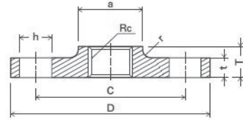
ねじ込みフランジ STF
