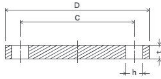
ブラインドフランジ BF
